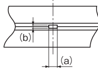
润滑孔的详细视图
